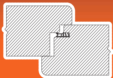
řez dveřma a zárubní
